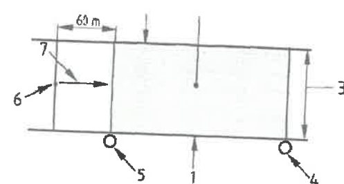
Figura 2: Stabilirea grilei de calcul pentru luminanta
