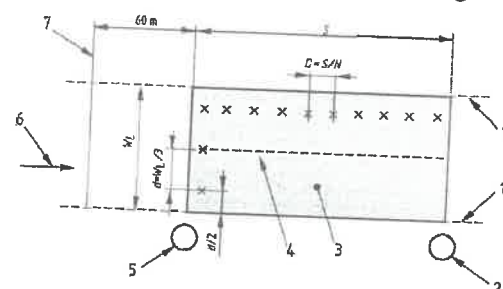
Figura 3: Poziția punctelor de calcul
