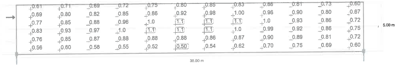
Observator 2: Densitatea luminii la instalația nouă [cd/m²] (Raster valoric)
