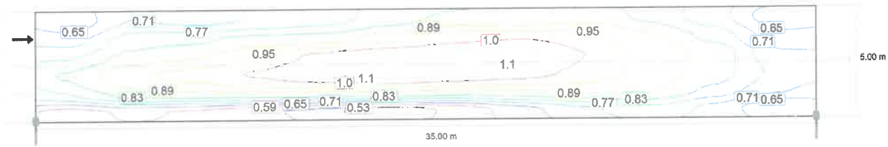
Observator 2: Densitatea luminii la instalația nouă [cd/m²] (Linii Isolux)
